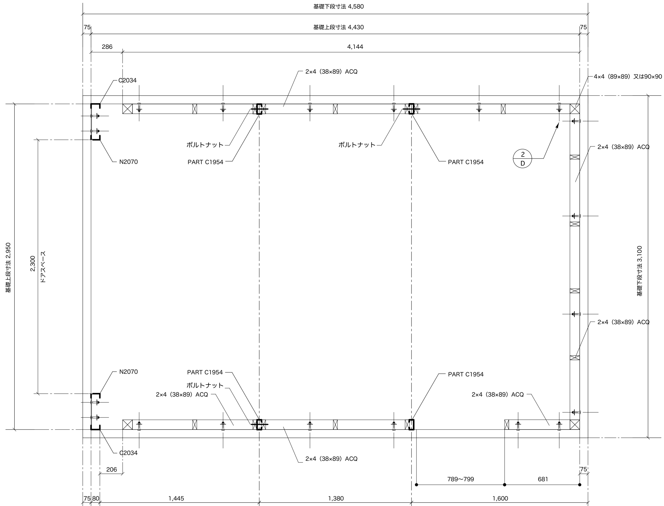
平面図（下枠材） 1/20
