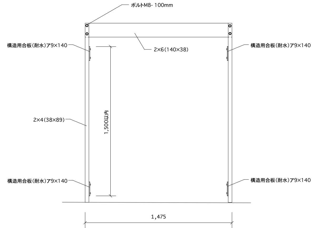
展開図 1/20 C-C
