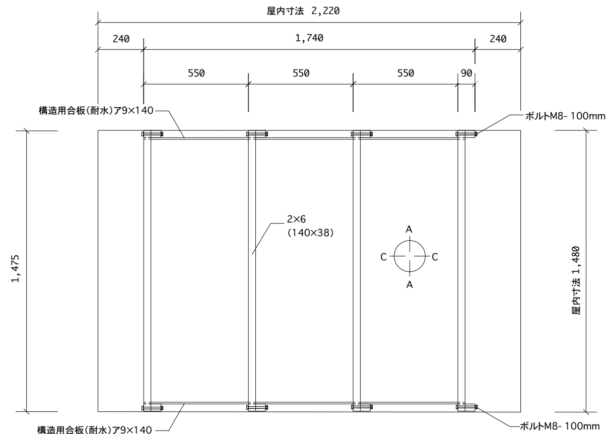
天井下図 1/20
