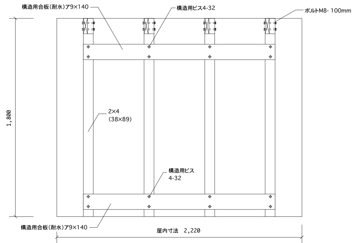
展開図 1/20
